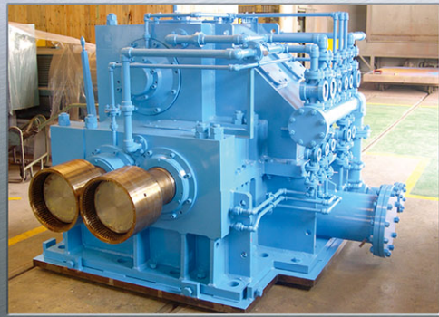
ミキシングローラー用歯車減速機 Mixing Roll Gear Reducer (1500 KW, 18 Tons)
