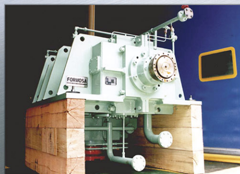
棒鋼ミル用ピニオンスタンド Vertical Reduction Pinion Stand for Bar Mill (500 KW, 10 Tons)
