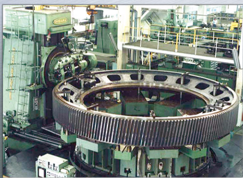
大型ホブ盤 (最大 7500mm) Ø7.5 Meter Precision Hobbing Machine
