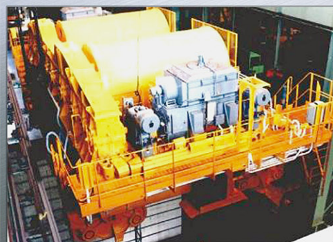
400 トンレードルクレーン用歯車減速機 Gear Reducer for 400 Tons Ladle Crane
