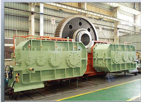
厚板用クロップシャー設備 Plate Mill Crop/Divide Shear Equipment (2 × 650 KW, 500 Tons)
