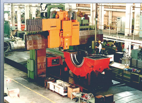
縦型ターニングマシン
