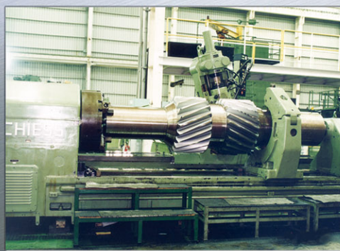
横型ホブ盤 (最大 1400mm、長さ 4000mm) Horizontal Type Hobbing Machine (Max Ø1.4 M × 4 ML)
