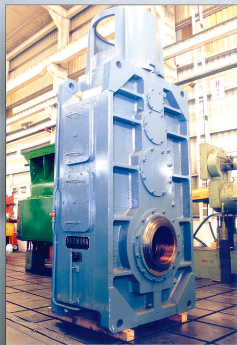
スタッカリクレーマ用歯車減速機 Stacker & Reclaimer Gear Reducer
