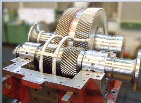
高速歯車増速機の組立 Assembly of High Speed Gear Increaser
