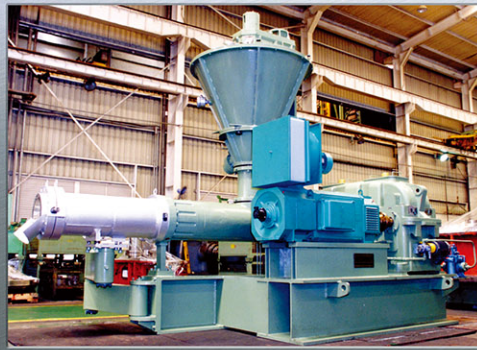
ペレット製造装置 メルト ポンプ用遊星歯車減速機 Planetary Gear Reducer for Melt Pump (650 KW, 7 Tons)
