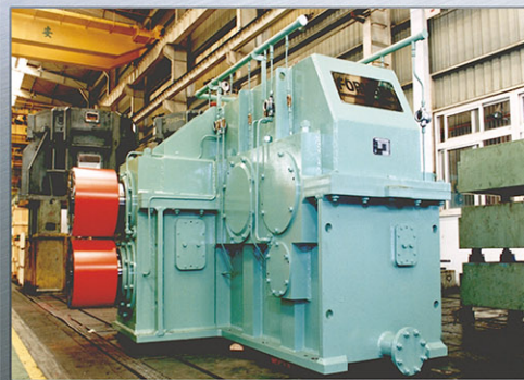
ビレットミル用ピニオンスタンド Horizontal Reduction Pinion Stand for Billet Mill (700 KW, 17.5 Tons)
