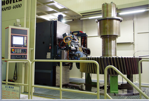
内歯・外歯用複合大型歯車研削盤 (最大 4000mm) Ø4.0 Meter Profile Gear Grinding Machine for External & Internal Gear
