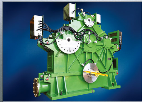
コンプレッサー用多段歯車箱 Integral Multi-stage Gearbox for Compressor
