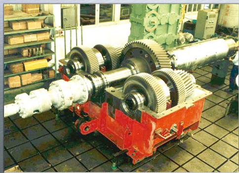
減速機の組立・歯当たり検査 Assembly & Contact Pattern Inspection
