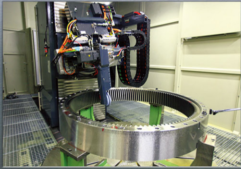
大型ホブ盤 (最大 7500mm) Ø7.5 Meter Precision Hobbing Machine
